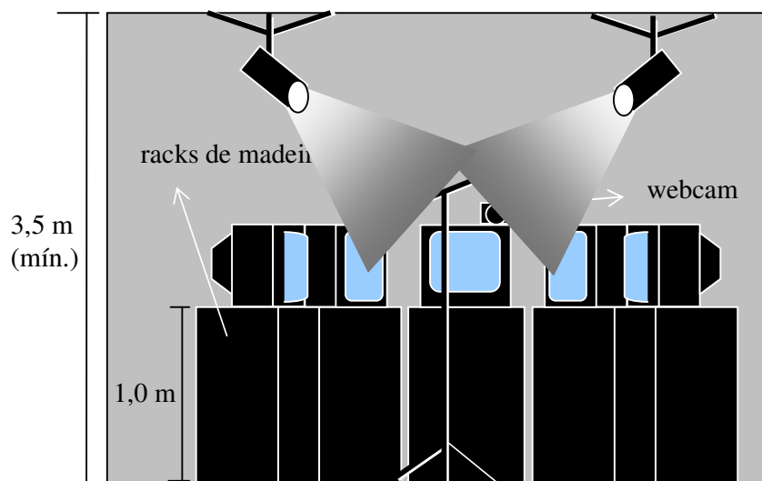
Figura 2 Vista frontal da instalação
