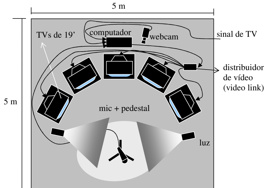
Figura 1 Vista superior da instalação
